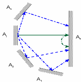
Abbildung 1: Einzeleinflüsse der Fläche A_j auf A_k für langwellige Strahlung
