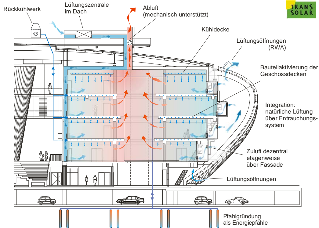
Abbildung 1: Schematische Darstellung des Klima- und Energiekonzepts für den Ausstellungsbereich Elemente im Sommerfall
