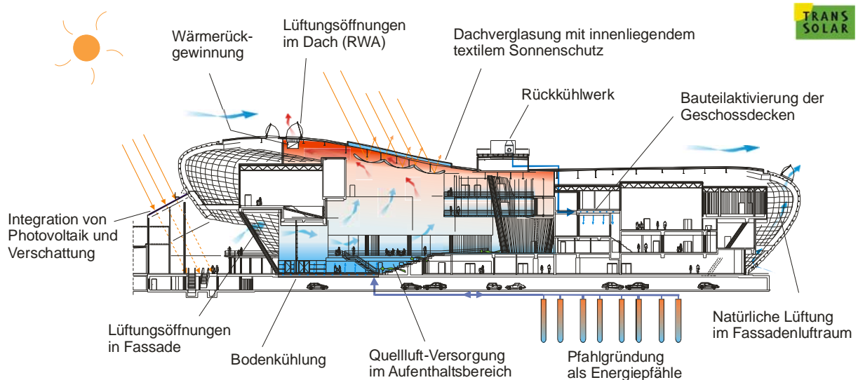
Abbildung 2: Schematische Darstellung einiger Elemente des Klima- und Energiekonzepts im Längsschnitt durch das Klimahaus®
